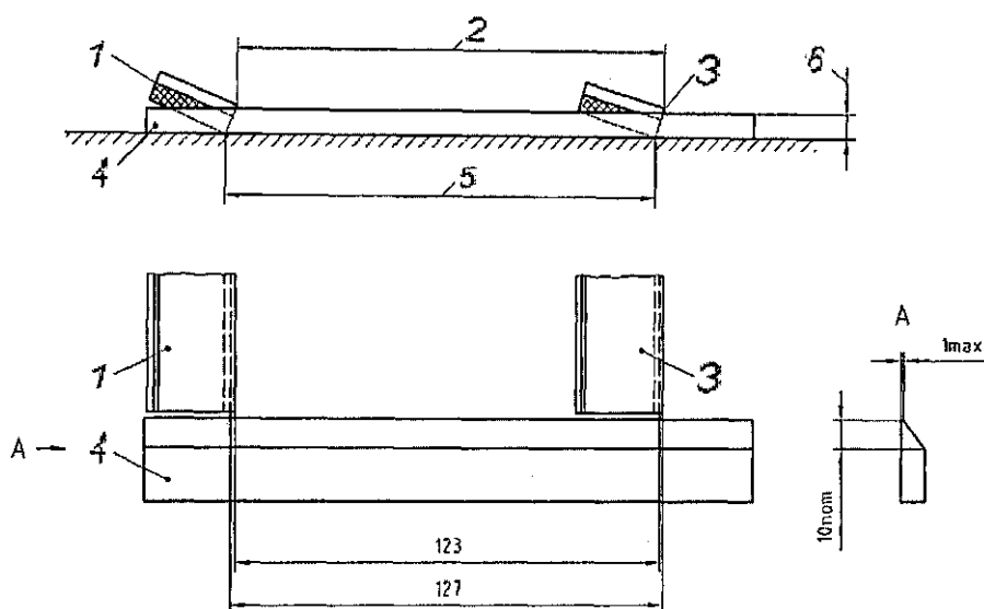
Рисунок 7. Устройство регулировки длины пятна контакта
